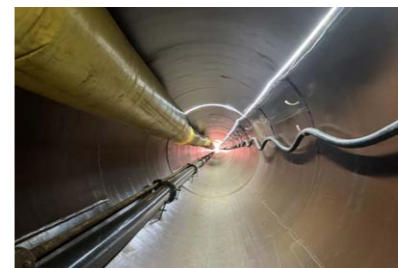
排海管工程
