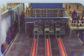
R8米3流立弯式连铸机
