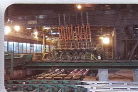
R8.5米6流连铸机
