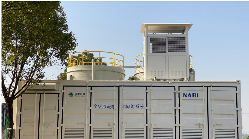
250kW_1MWh 全钒液流电池储能电站应用于湖北省能源互联网示范工程
